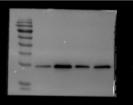
IL-6
