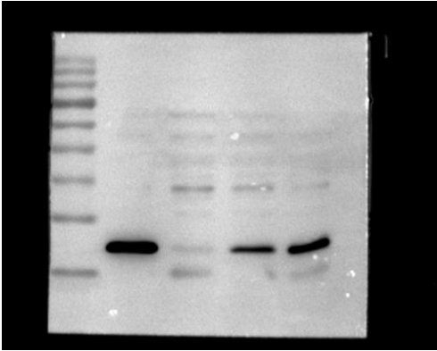
GPX4
