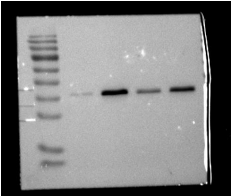
TNF-α
