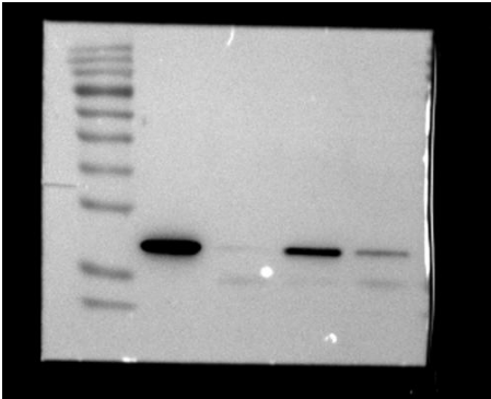
GPX4
