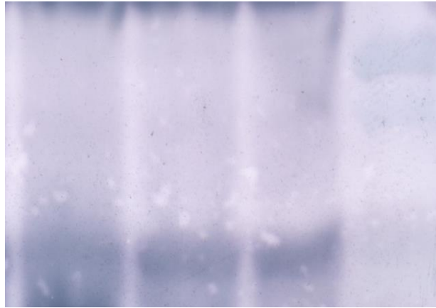
LSD1
