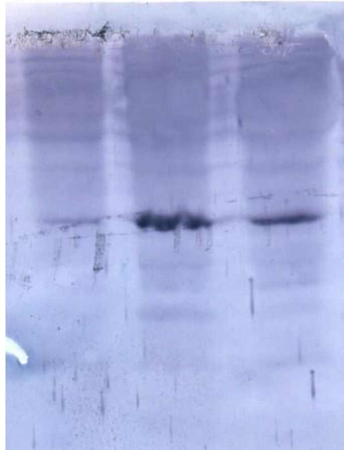
JARID2
