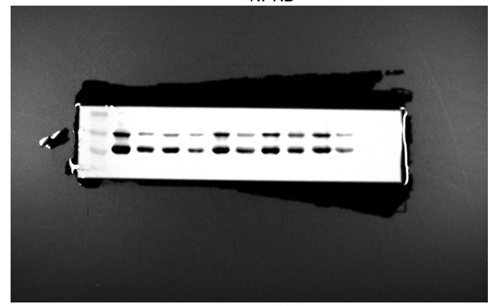
JNK
