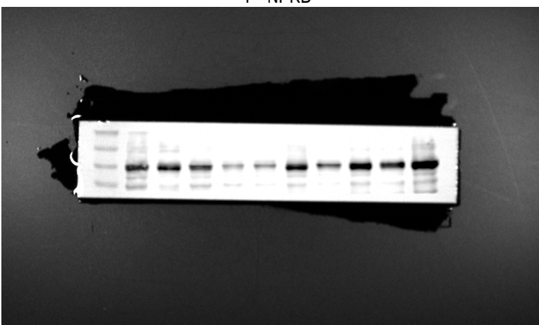
P-JNK
