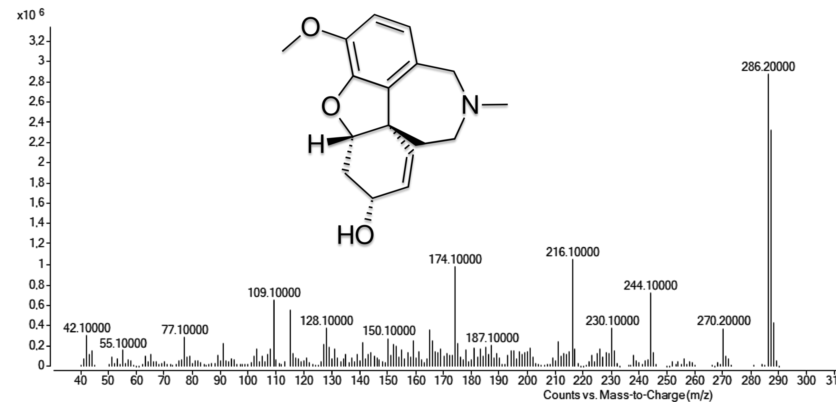
GC-MS
