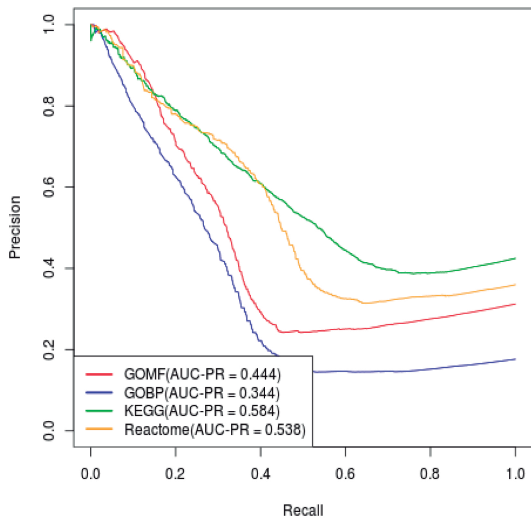
(d) Jaccard
