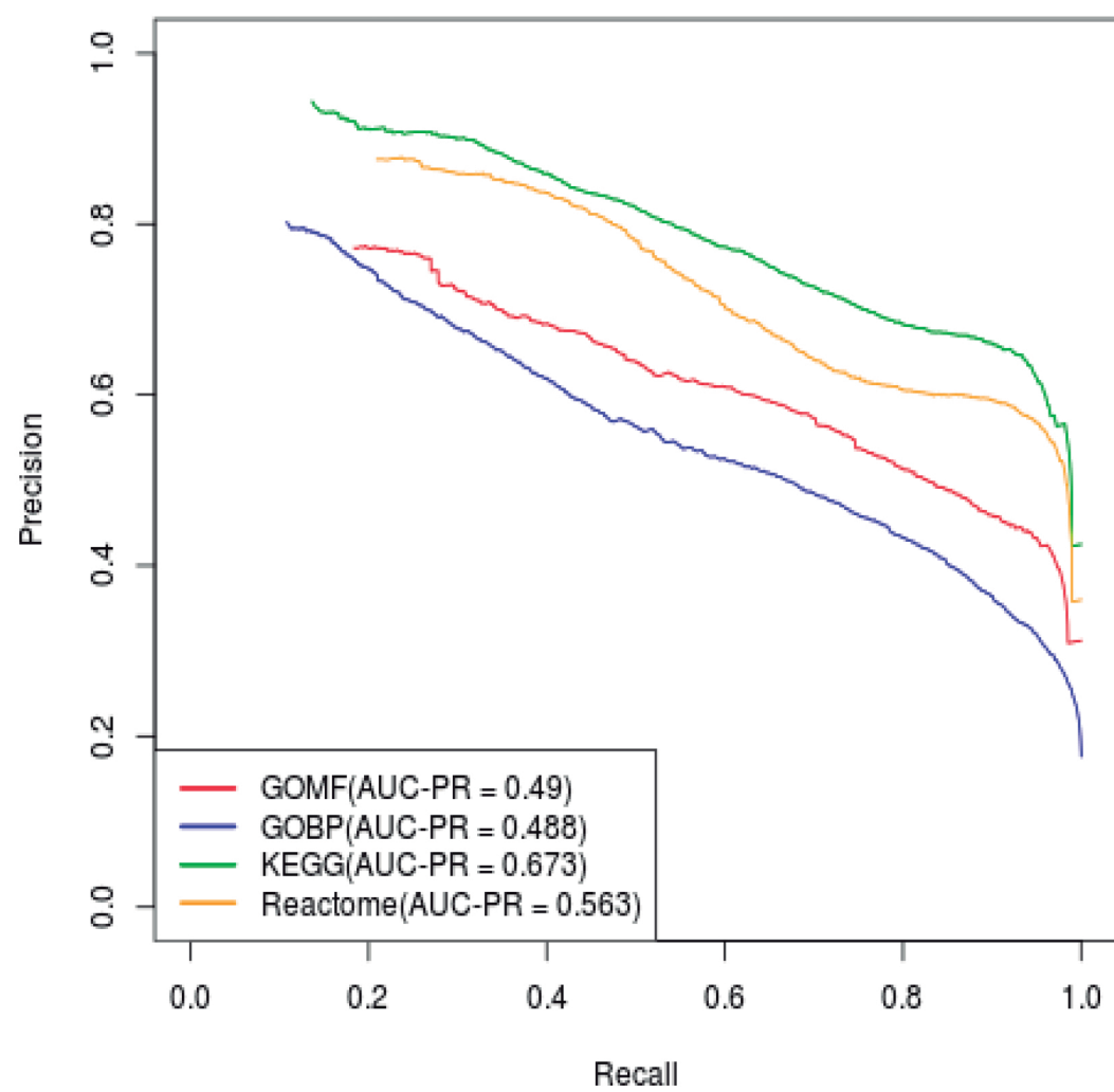
(f) HyI
