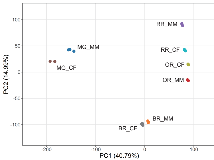
2D PCA Plot
