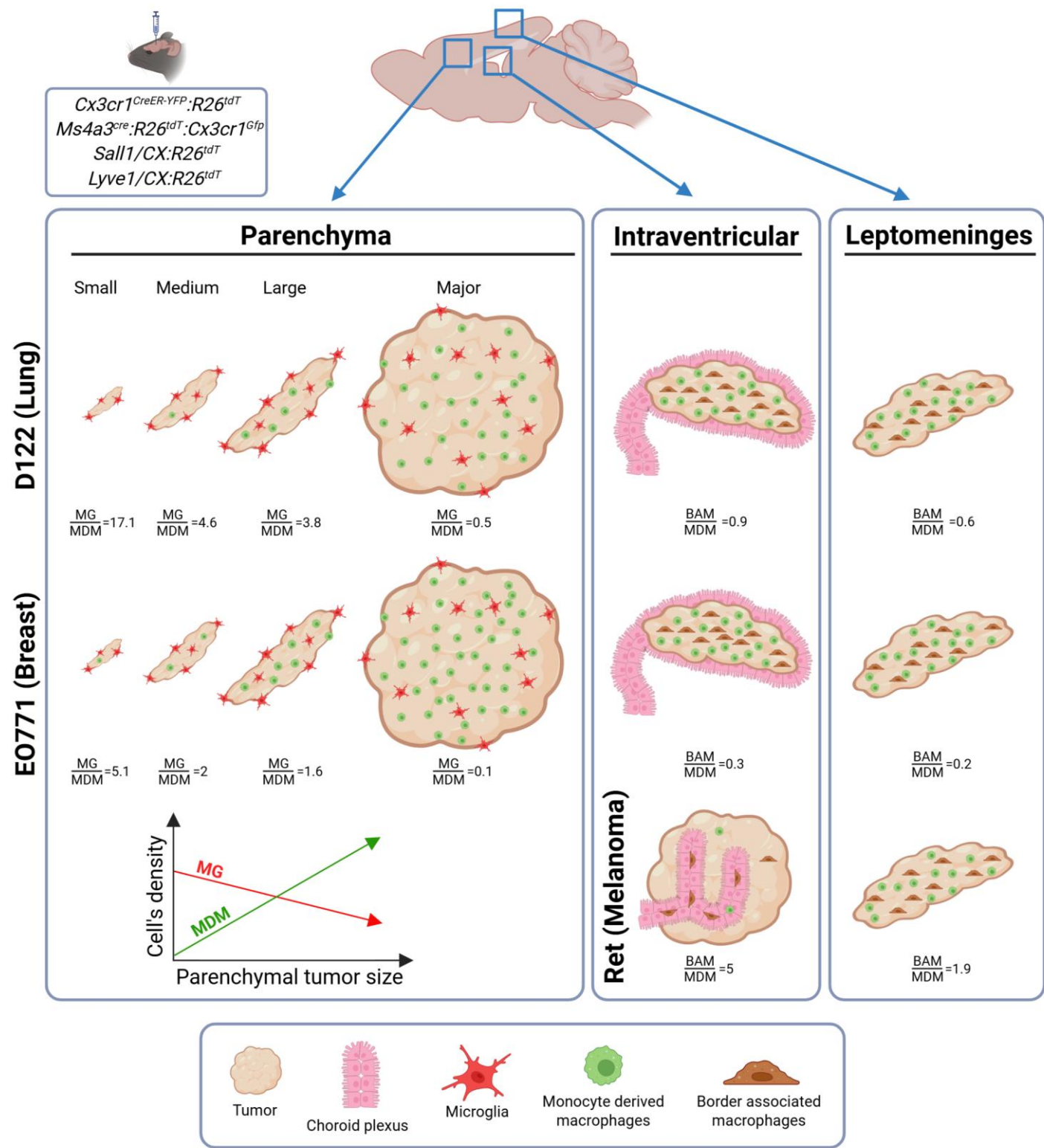
Fig. S13
