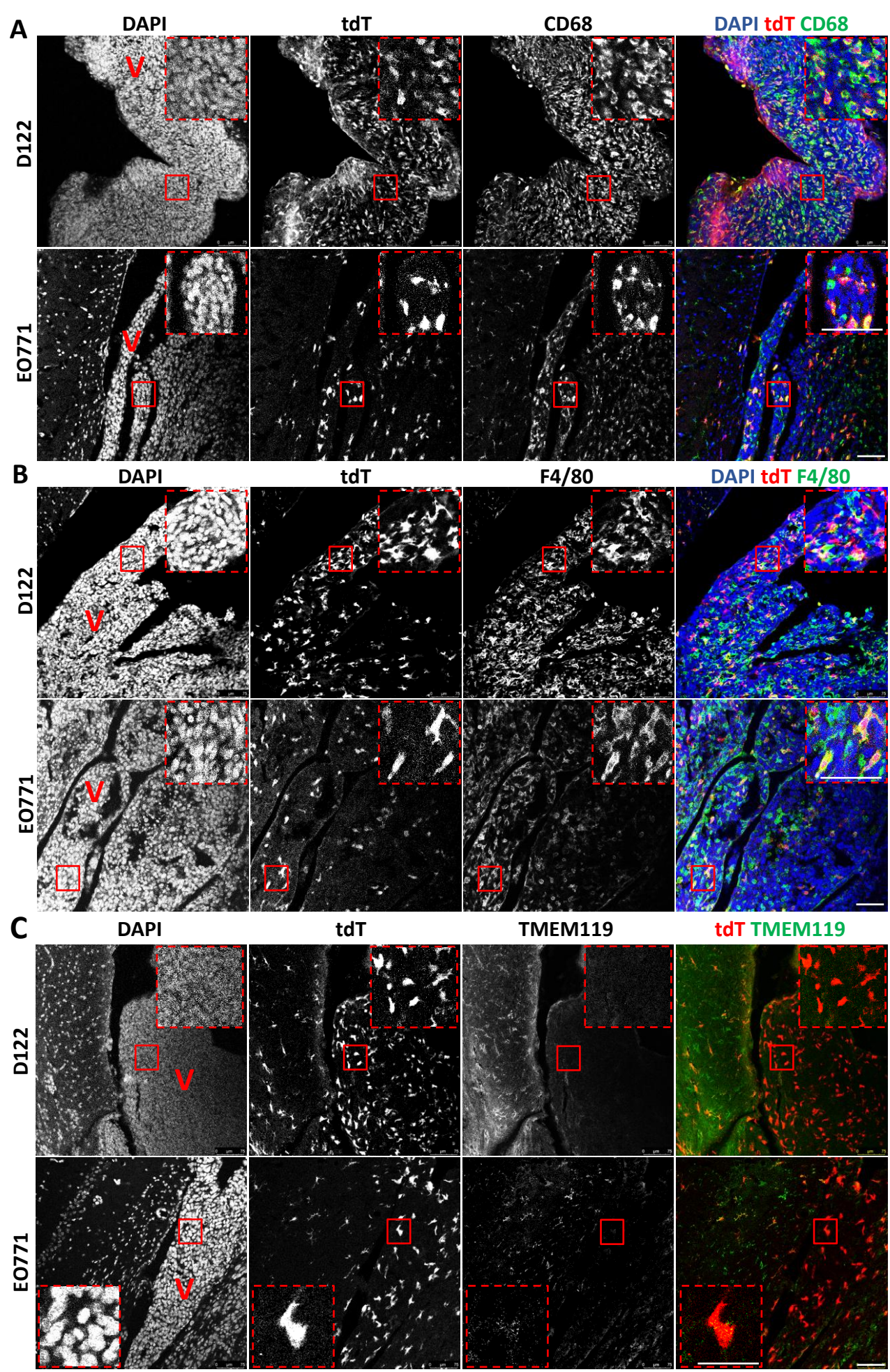
Fig. S10
