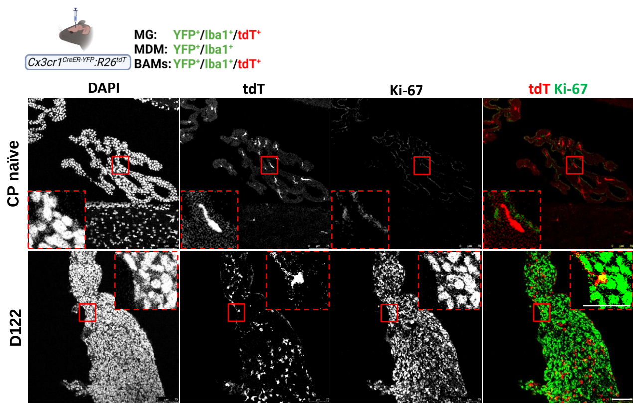
Fig. S9
