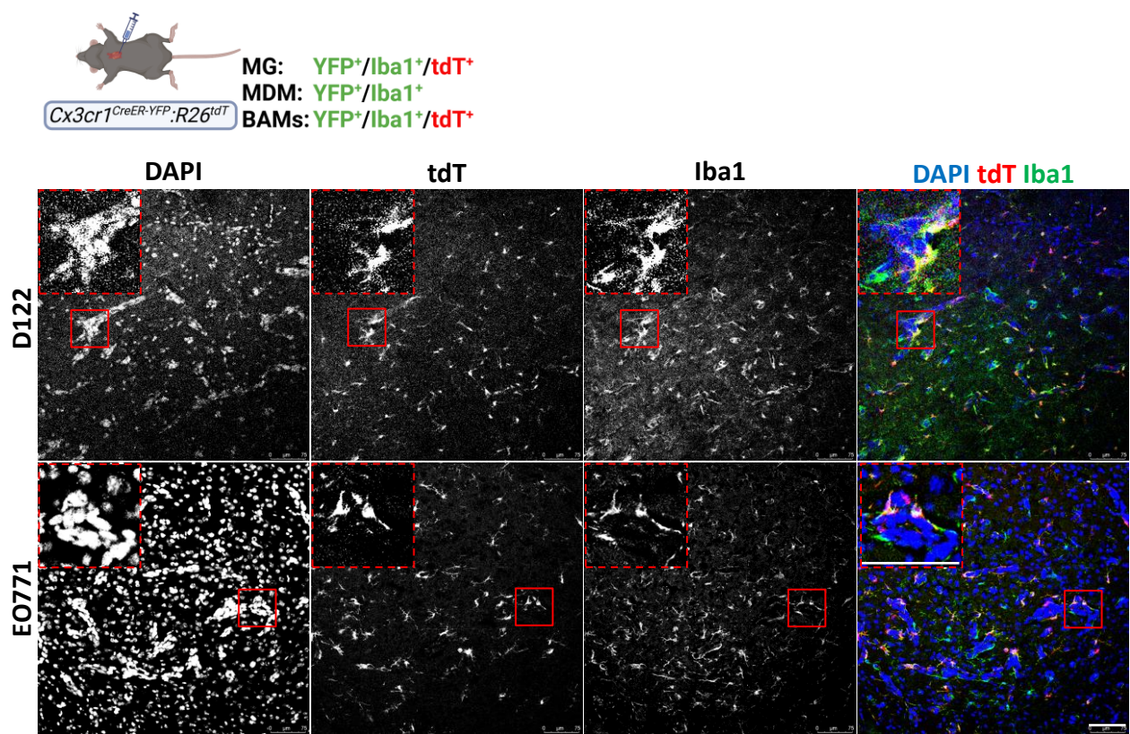
Fig. S8
