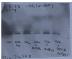
ID4
