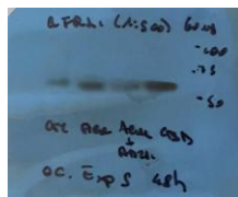
GFRA1
