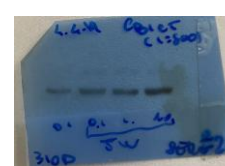
CB1
