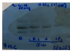
MAGL
