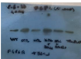
FGF2
