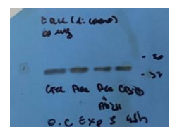
ERK
