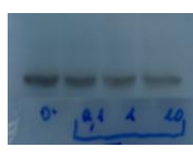
MAGL
