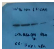
ID4
