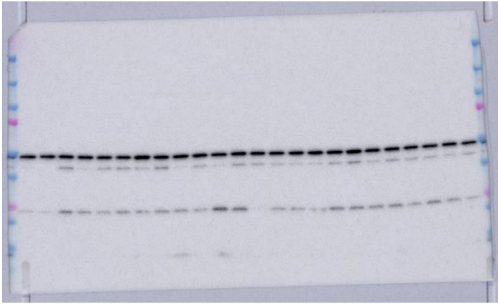
INSIG2
