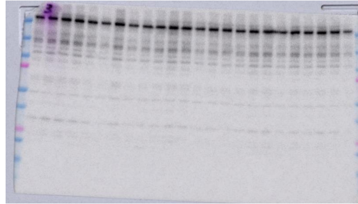
FAS
