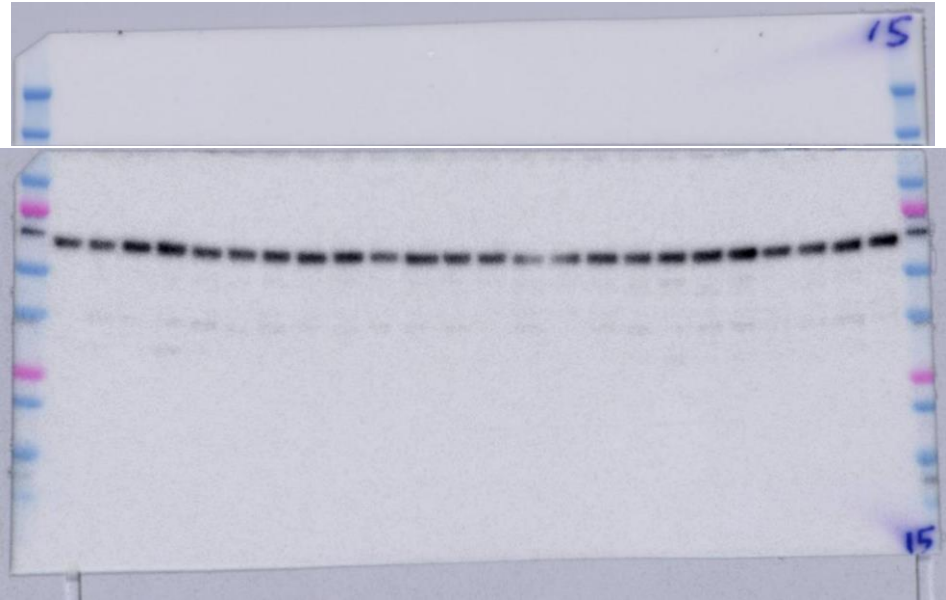
PPAR \gamma
