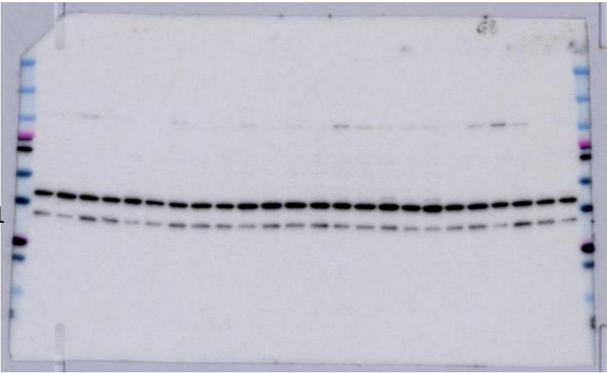
USF1
