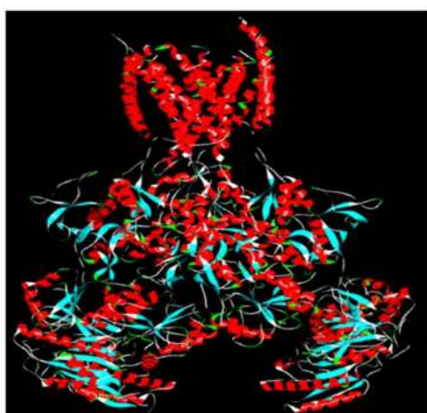
6IRH
