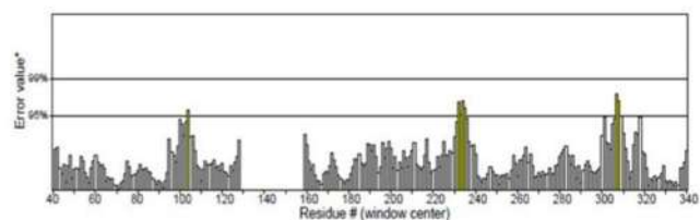
ERRAT
