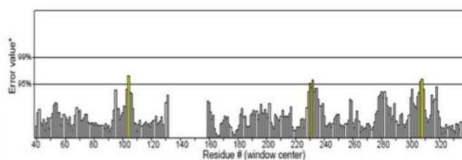
ERRAT
