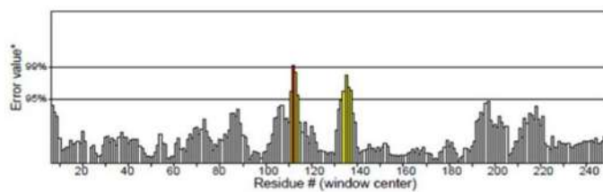
ERRAT
