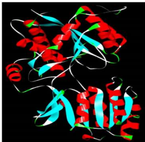
2WJW
