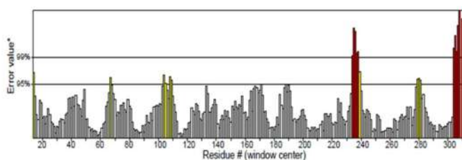
ERRAT
