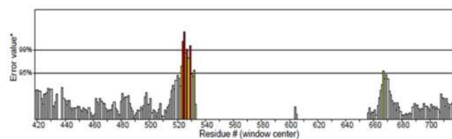
ERRAT
