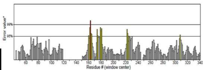
ERRAT
