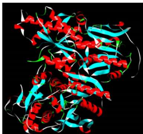
6BSZ
