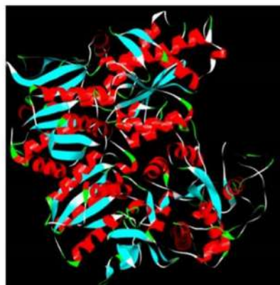
1EWK
