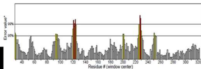
ERRAT
