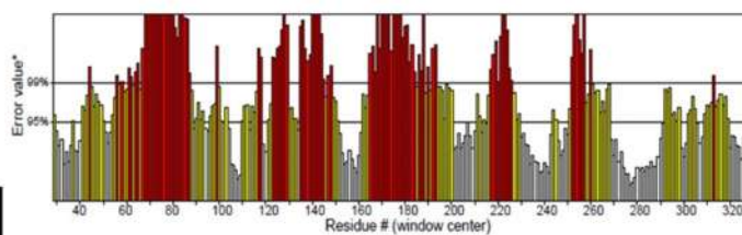
ERRAT
