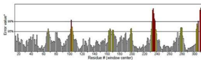
ERRAT
