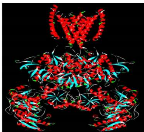
7EOR
