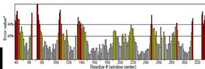
ERRAT
