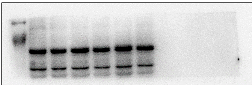
Fig E-AMPK
