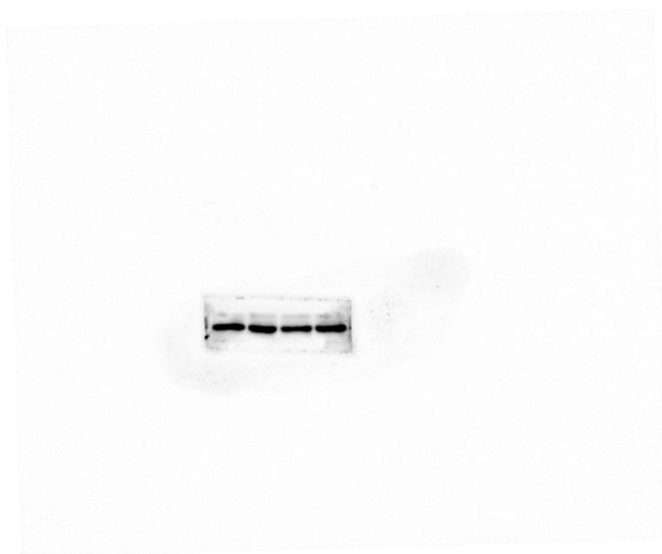
PFK1-A549
