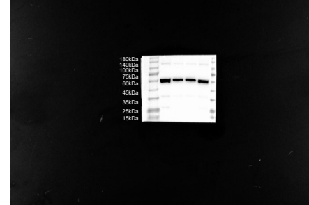
ACSL4
