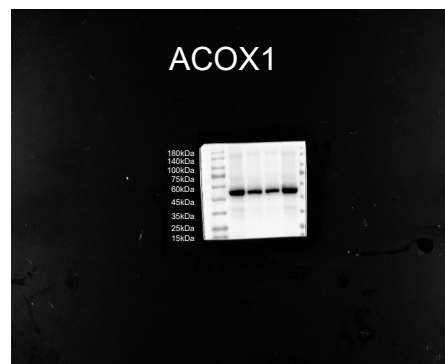
MDA-MB-231
