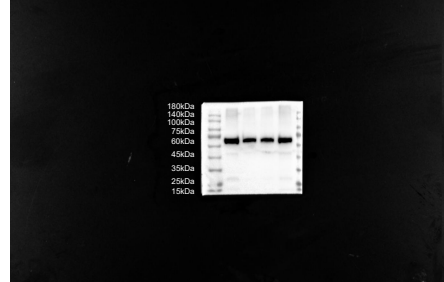
ABCD3
