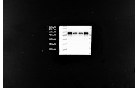
EHHADH
