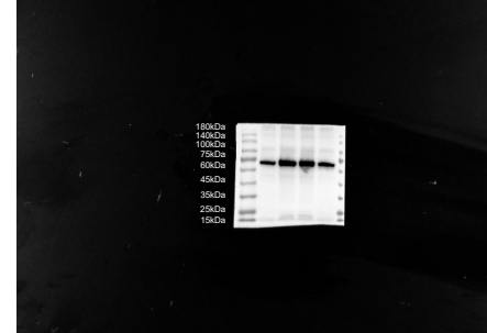
ACSL4
