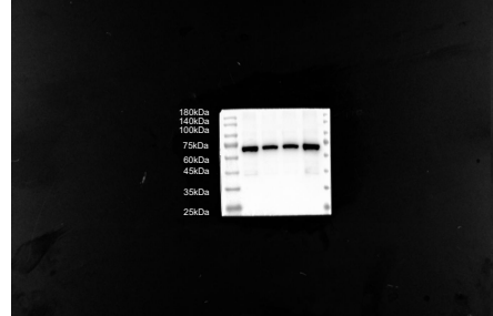
ABCD4
