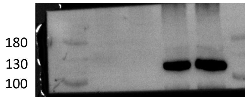
iNOS 120kDa
