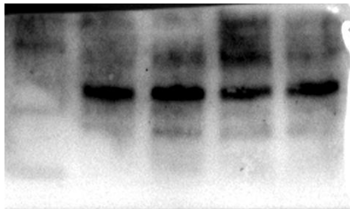
ARG1 35kDa
