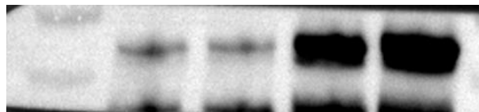
Akt 56kDa
