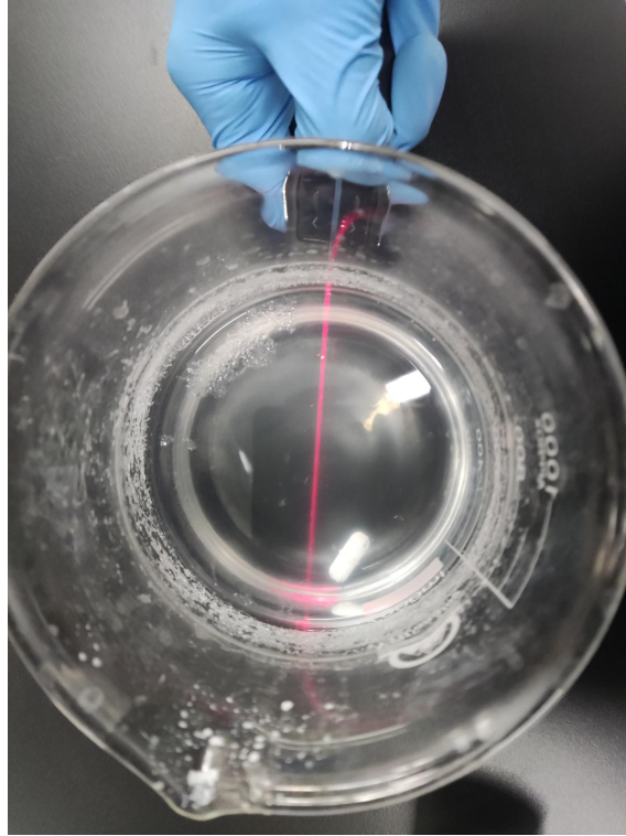
Fig.1 \text{SiO}_2 sol
