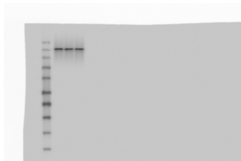
LRP6
