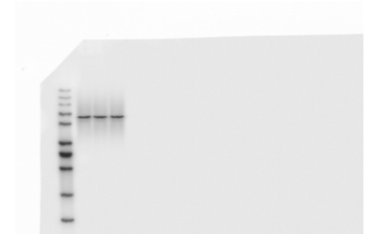
Dvl3
