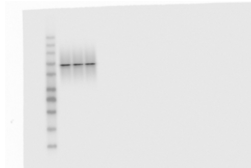
Dvl2
