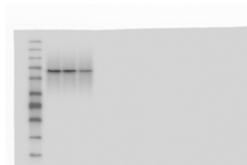
Dvl3
