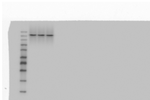
LRP5
