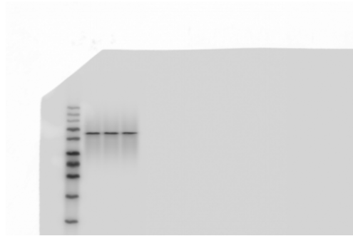
Dvl1
