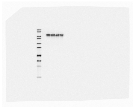
IP-Axin1-IB-Axin1
