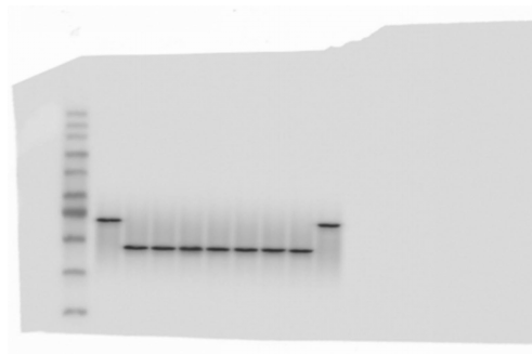
input-HA
