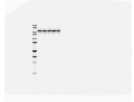
input-Axin1
