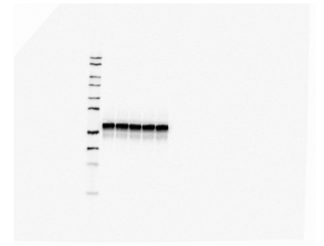
input-β-actin
