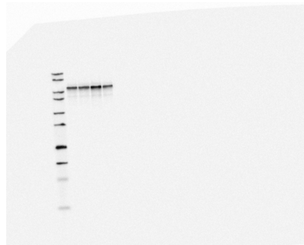
Axin1
