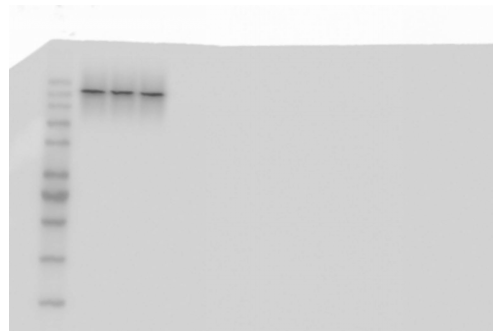
input-Flag
