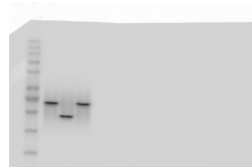
input-HA
