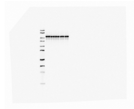
input-Axin1
