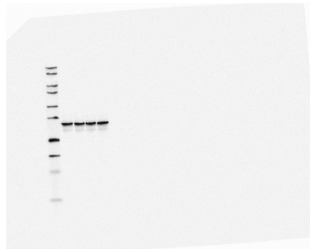
p-GSK3β (Ser9)
