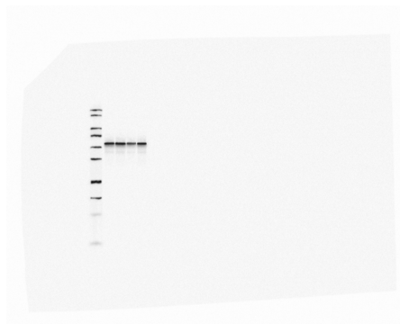
membrane Dvl1
