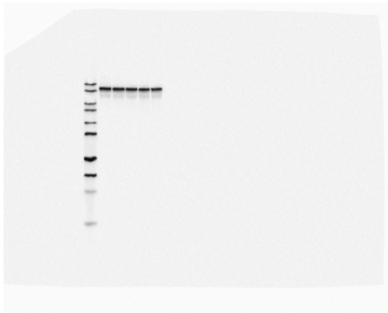
input-APC
