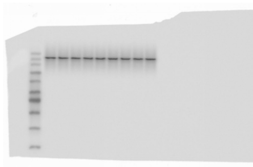
input-Flag
