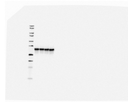
GSK3β
