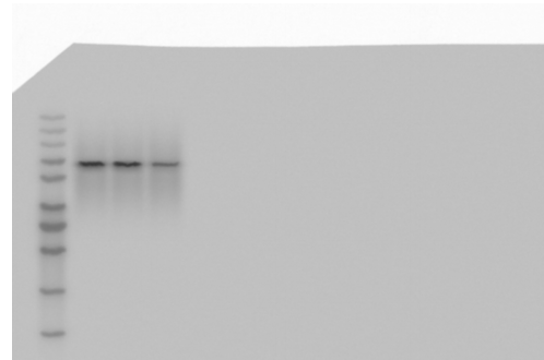
membrane Dvl2
