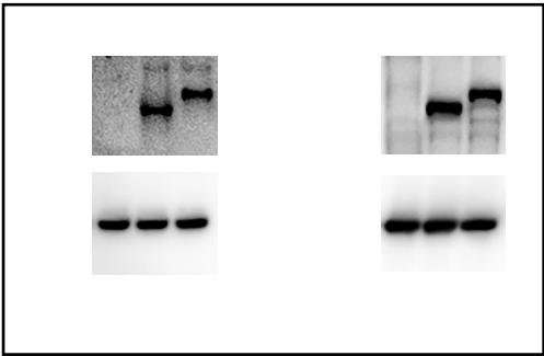
A2780/KD
