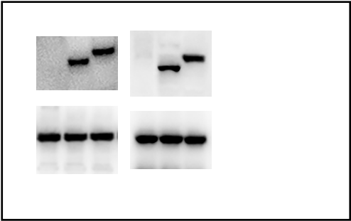
SKOV3/KD
