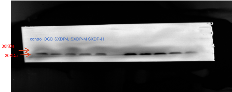
GPx1
