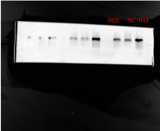
DNMT1
