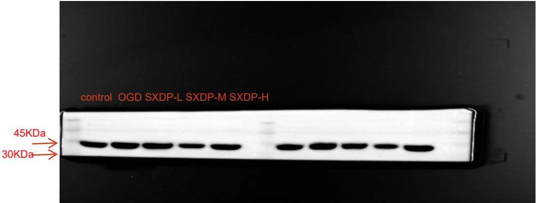
IL-1 \beta
