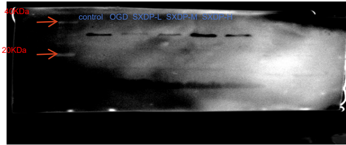
SOD
