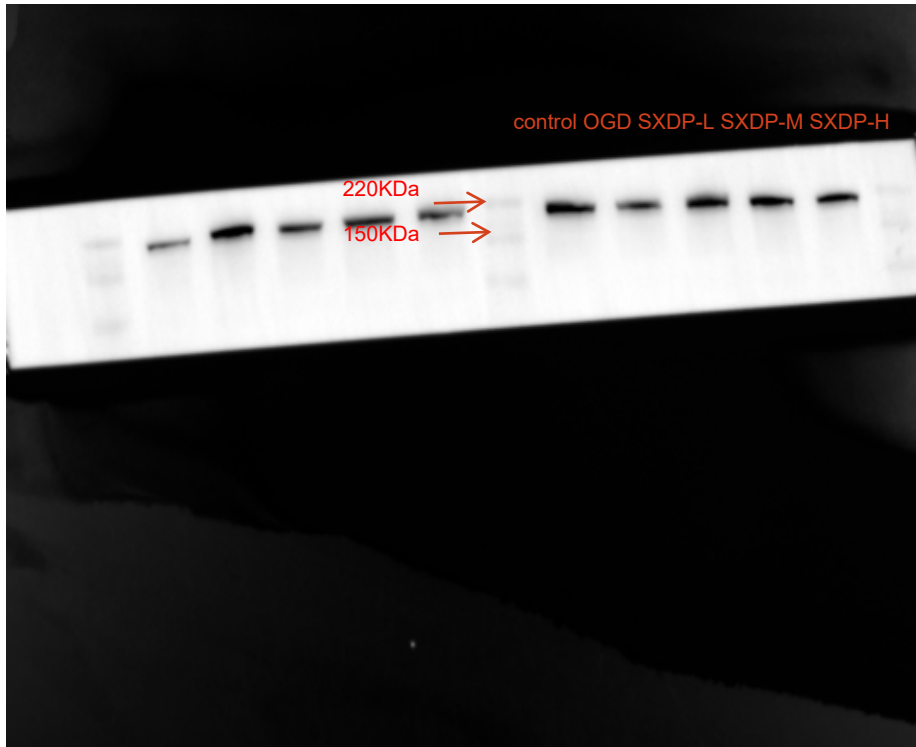
DNMT1
