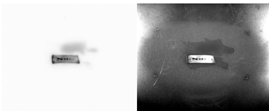
RT4 Rad51
