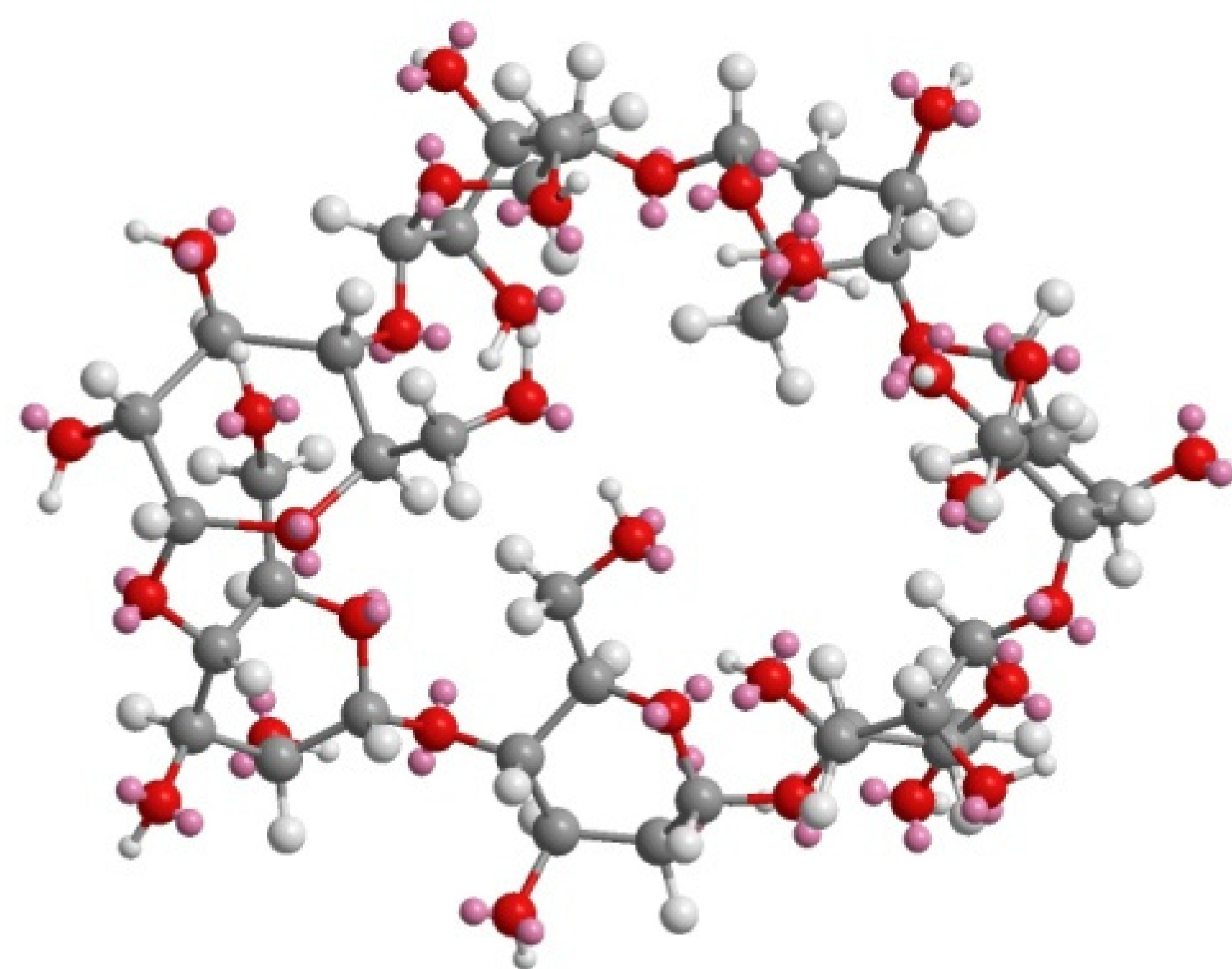
\beta -Cyclodextrin ( \beta -CD)
