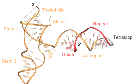
CjCas9 (PDB: 5X2G)
