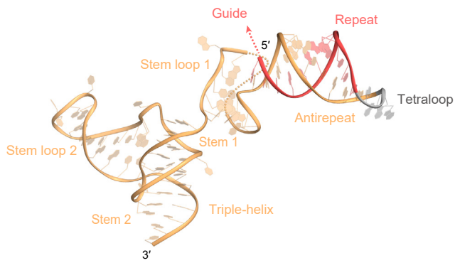
SaCas9 (PDB: 5CZZ)
