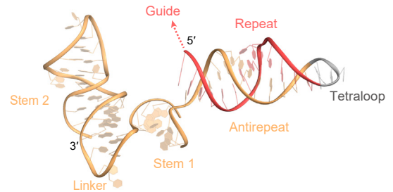
FnCas9 (PDB: 5B2O)
