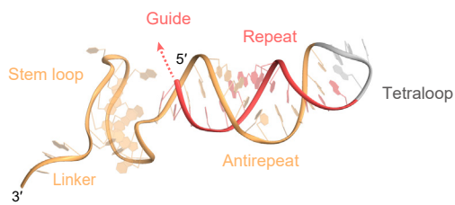
SaCas9 (PDB: 5CZZ)
