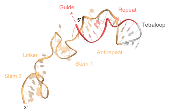
FnCas9 (PDB: 5B2O)
