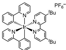
PC 3: [Ir(ppy) 2 (dtbbpy)]PF 6 c Ir III /Ir II = + 0.66 V Ir II /Ir III = - 1.51 V
