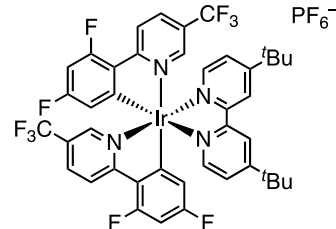
PC 4: [Ir(dF(CF 3 )ppy) 2 (dtbbpy)]PF 6 c Ir III /Ir II = + 1.21 V Ir II /Ir III = - 1.37 V
