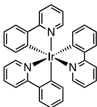
PC 2: fac -Ir(ppy) 3 c Ir III /Ir II = + 0.31 V Ir II /Ir III = - 2.19 V
