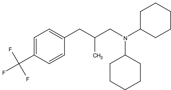
(±)-24 19 F NMR, 471 MHz, CDCl 3
