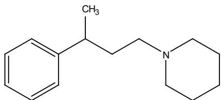
49 1 H NMR, 500 MHz, CDCl 3
