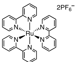
PC 1: [Ru(bpy) 3 ](PF 6 ) 2 c Ru III /Ru I = + 0.77 V Ru I /Ru II = - 1.33 V
