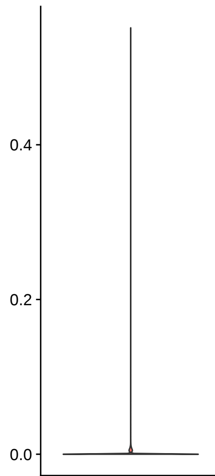
percent.HB
