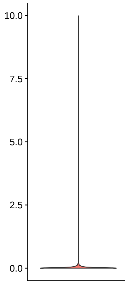
percent.HB
