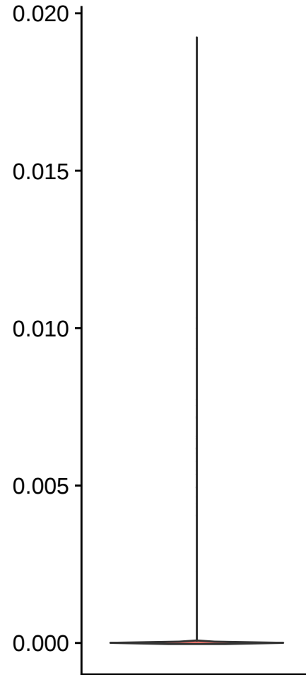
percent.HB
