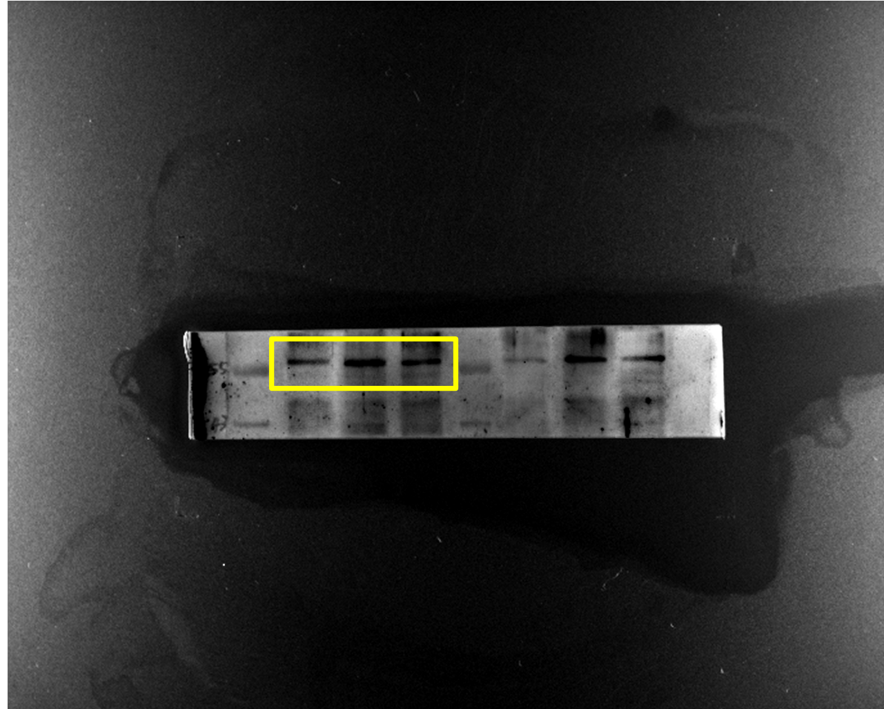
Acrolein--56KD
