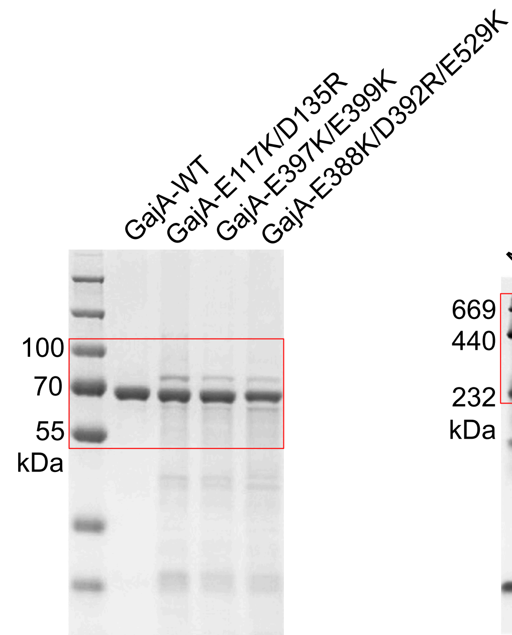
Extended Data Fig. 3b SDS-PAGE
