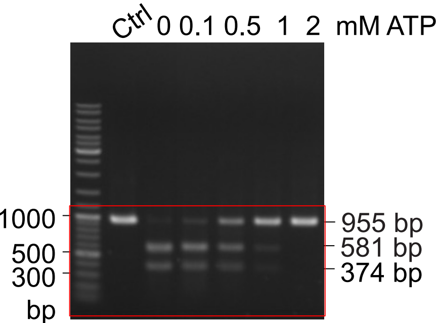
Extended Data Fig. 10a Titration of ATP
