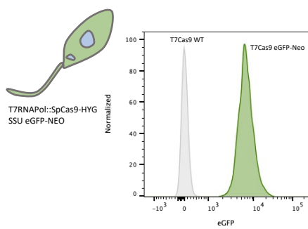
P L. tropica MA37
