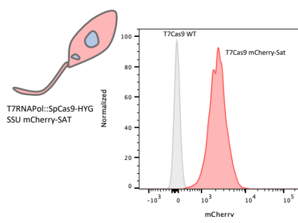
Q L. tropica L747
