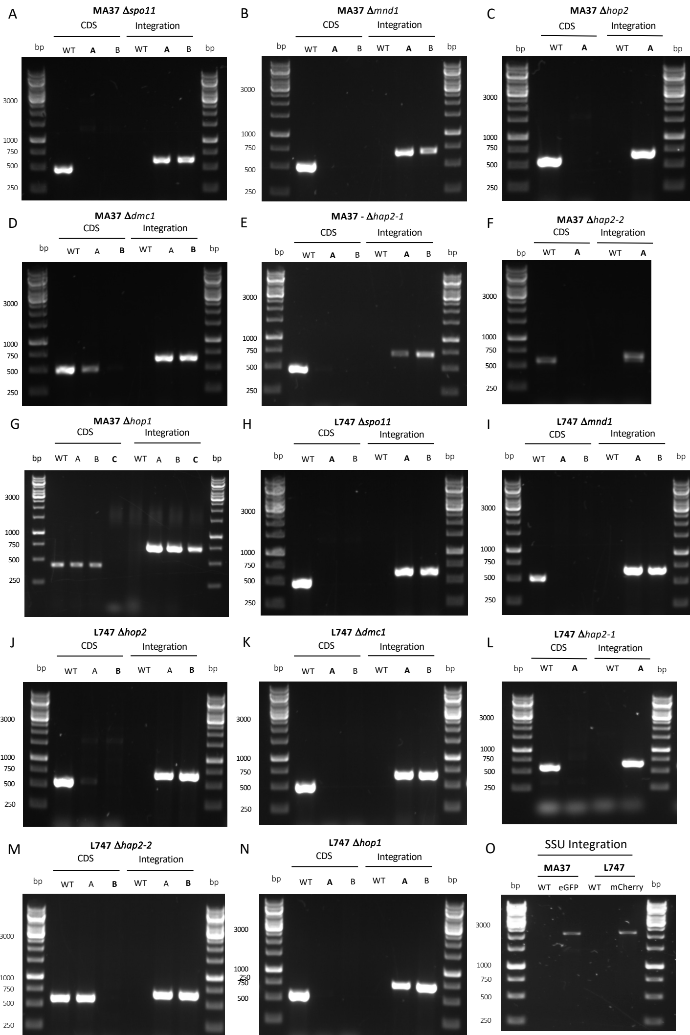
P L. tropica MA37
