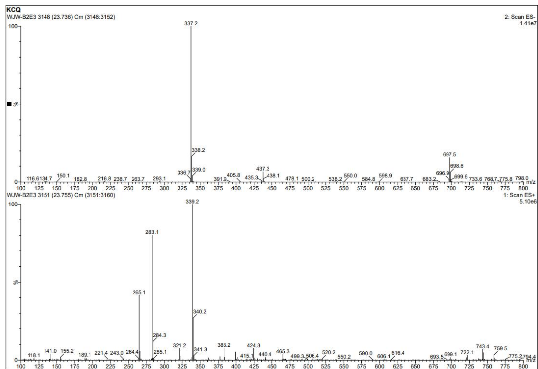
Fig. S3. The HRMS spectrum of CSA
