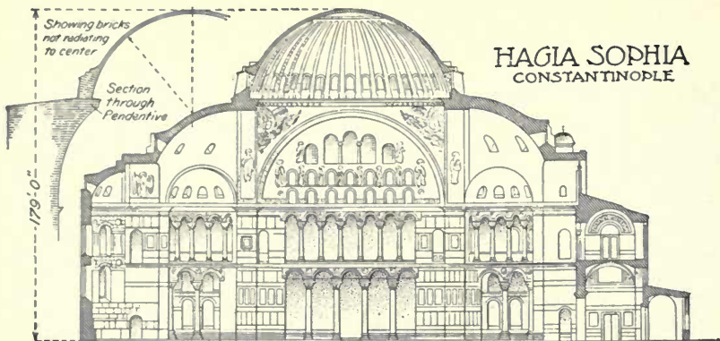
LONGITUDINAL SECTION
