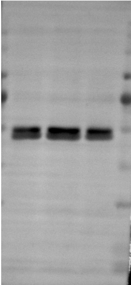
P-Akt
