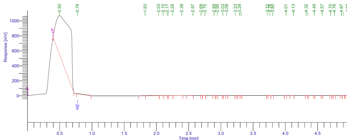
Fig. S3. GC of pure \text{H}_2 gas.
