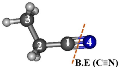
Propionitrile
