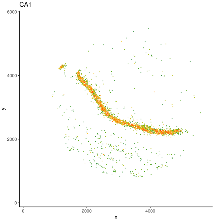
RCTD
