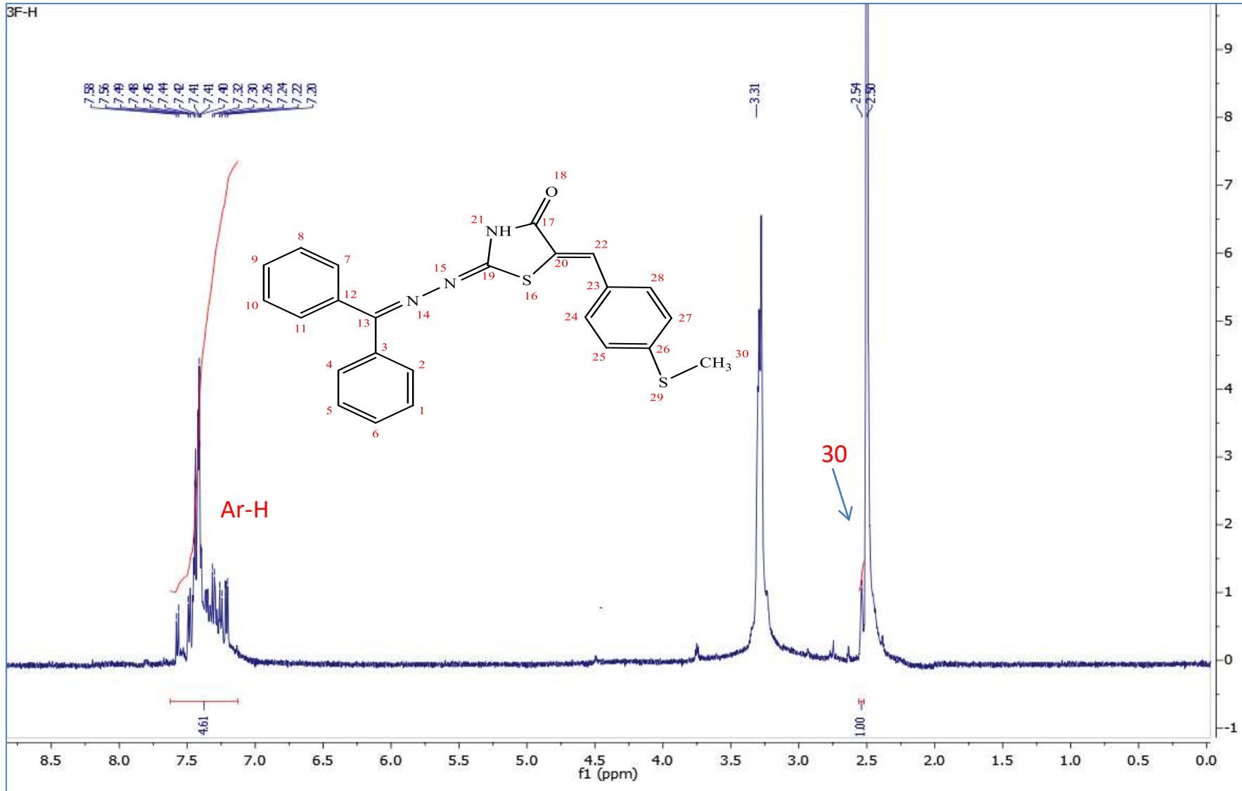
1H NMR spectrum of compound 3e
