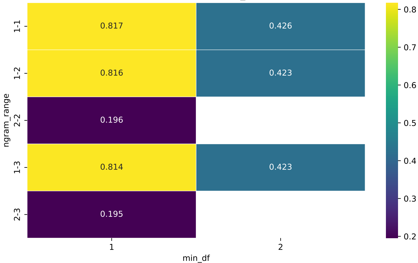
TF-IDF Mean MRR (sublinear_tf=False)
