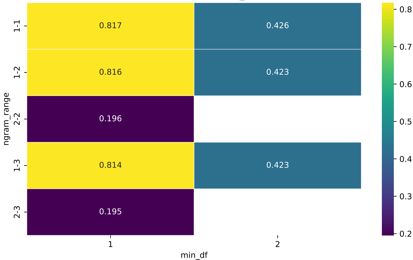
TF-IDF Mean MRR (sublinear_tf=True)
