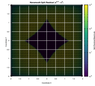
(d) 3D Obstacle Problem error a snapshot splitting method nonsmooth case
