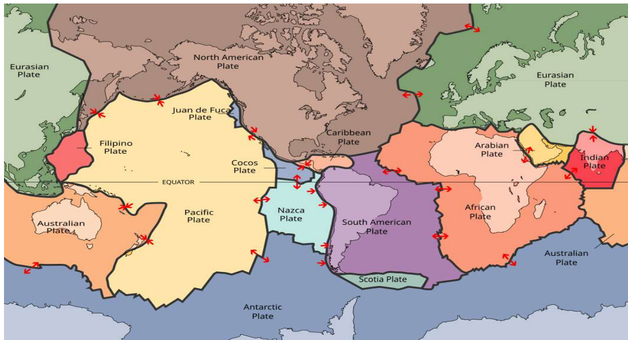
Рис.4. Map:USGS Description:Scott Nash, Tectonic plates.png
