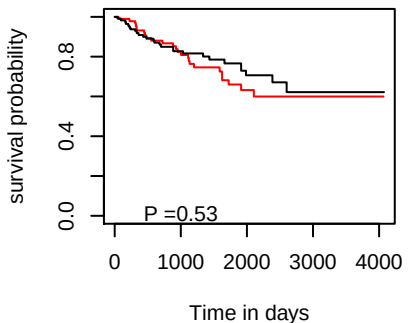
DSS hsa-mir-4742
