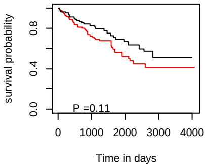
OS hsa-mir-320b-2
