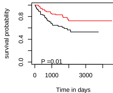
DSS hsa-mir-194-1
