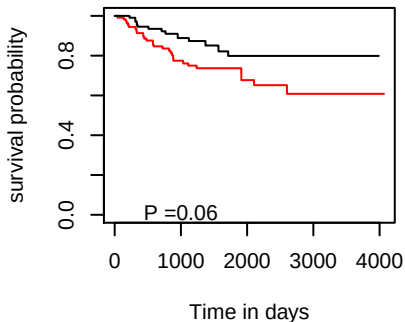
DSS hsa-mir-320b-2
