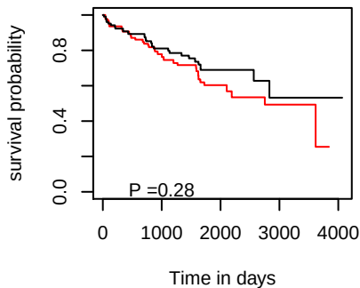
OS hsa-mir-4709
