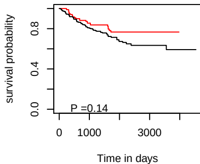
DSS hsa-mir-3131
