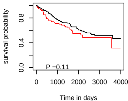
OS hsa-mir-4786
