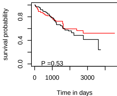
OS hsa-mir-2355
