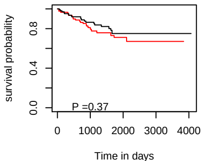
DSS hsa-mir-4709
