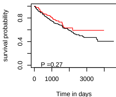
OS hsa-mir-3131
