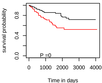
DSS hsa-mir-153-1
