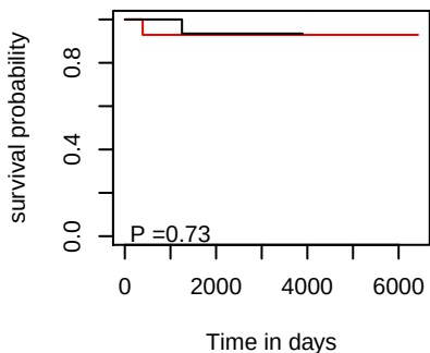
DSS hsa-mir-4773-2
