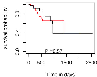
DSS hsa-mir-4664
