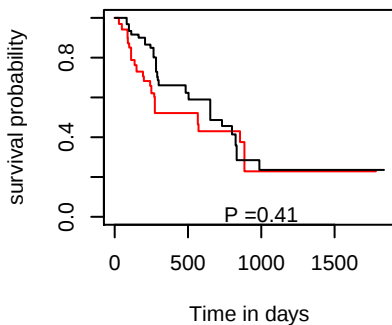
PFI hsa-mir-30e
