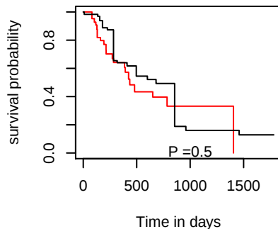
OS hsa-mir-548o
