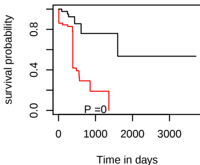
DSS hsa-mir-34c
