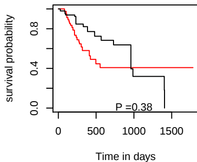
OS hsa-mir-4786
