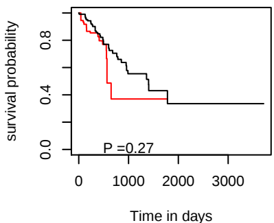
DSS hsa-mir-5687
