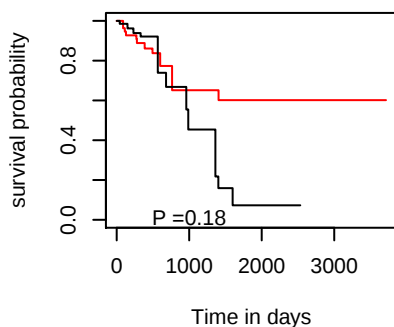
DSS hsa-mir-937
