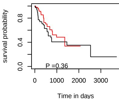
OS hsa-mir-3187
