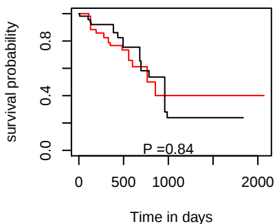
DSS hsa-mir-31
