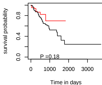
DSS hsa-mir-4691
