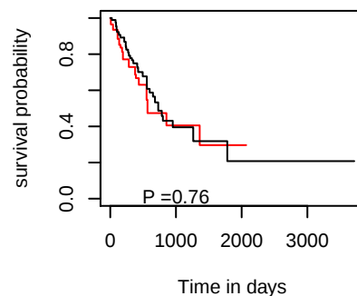
OS hsa-mir-4491
