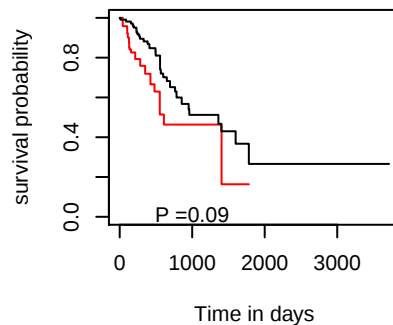
DSS hsa-mir-346
