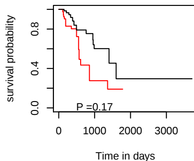
DSS hsa-mir-9-3
