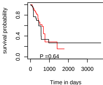
OS hsa-mir-491
