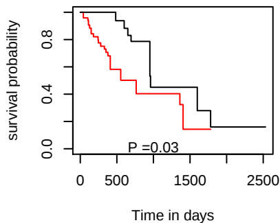
DSS hsa-mir-3648
