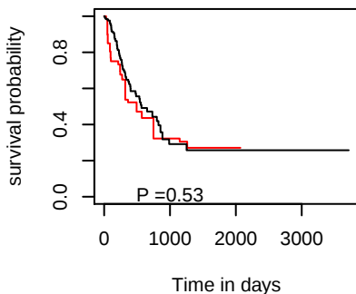
PFI hsa-mir-548t
