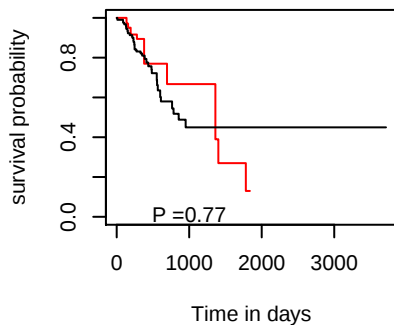
DSS hsa-mir-5703
