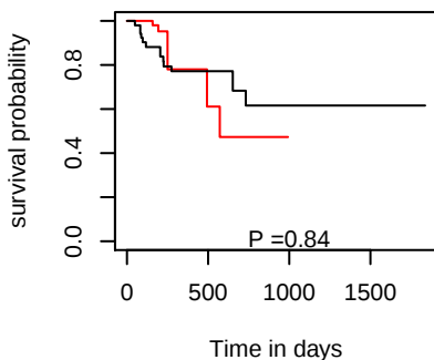
DFI hsa-mir-548d-1
