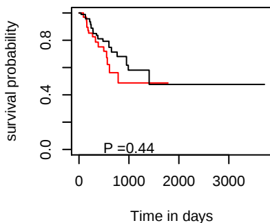
DSS hsa-mir-4444-2
