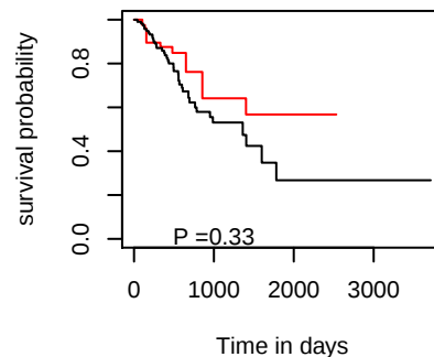
DSS hsa-mir-4529
