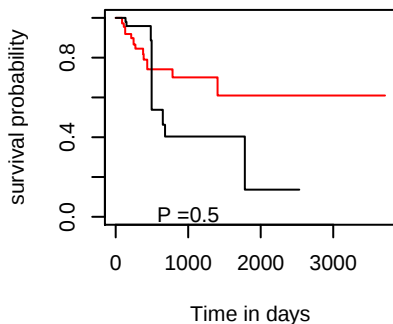
DSS hsa-mir-151a
