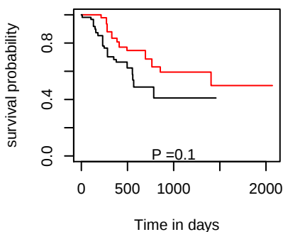
DSS hsa-mir-3691
