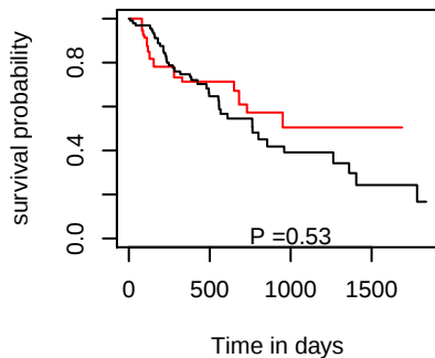
OS hsa-mir-4658
