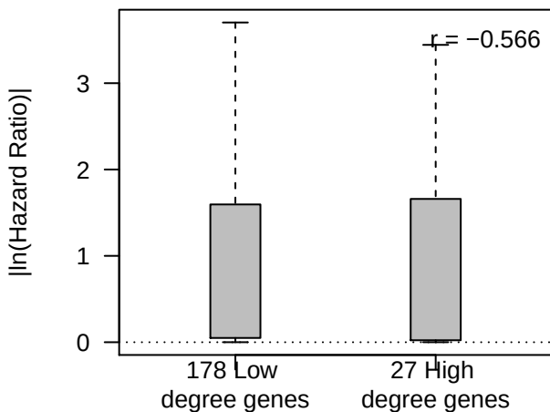
LUSC OS
