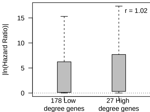
LUSC DSS
