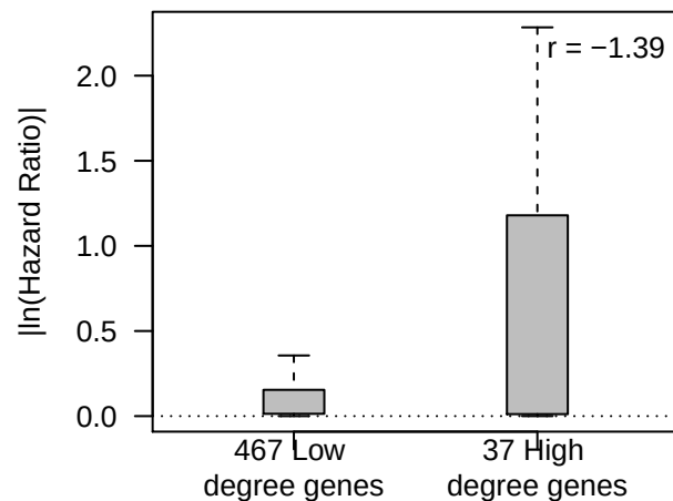
LUAD DFI
