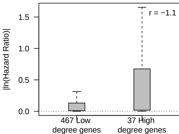
LUAD DSS
