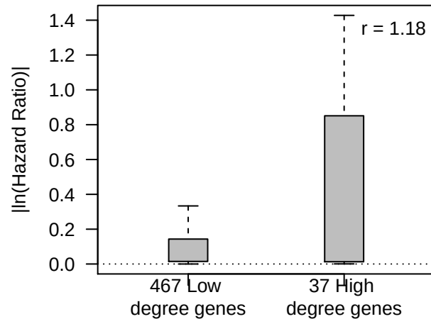
LUAD PFI
