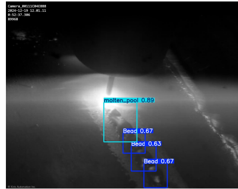
(d) Molten and Bead detection
