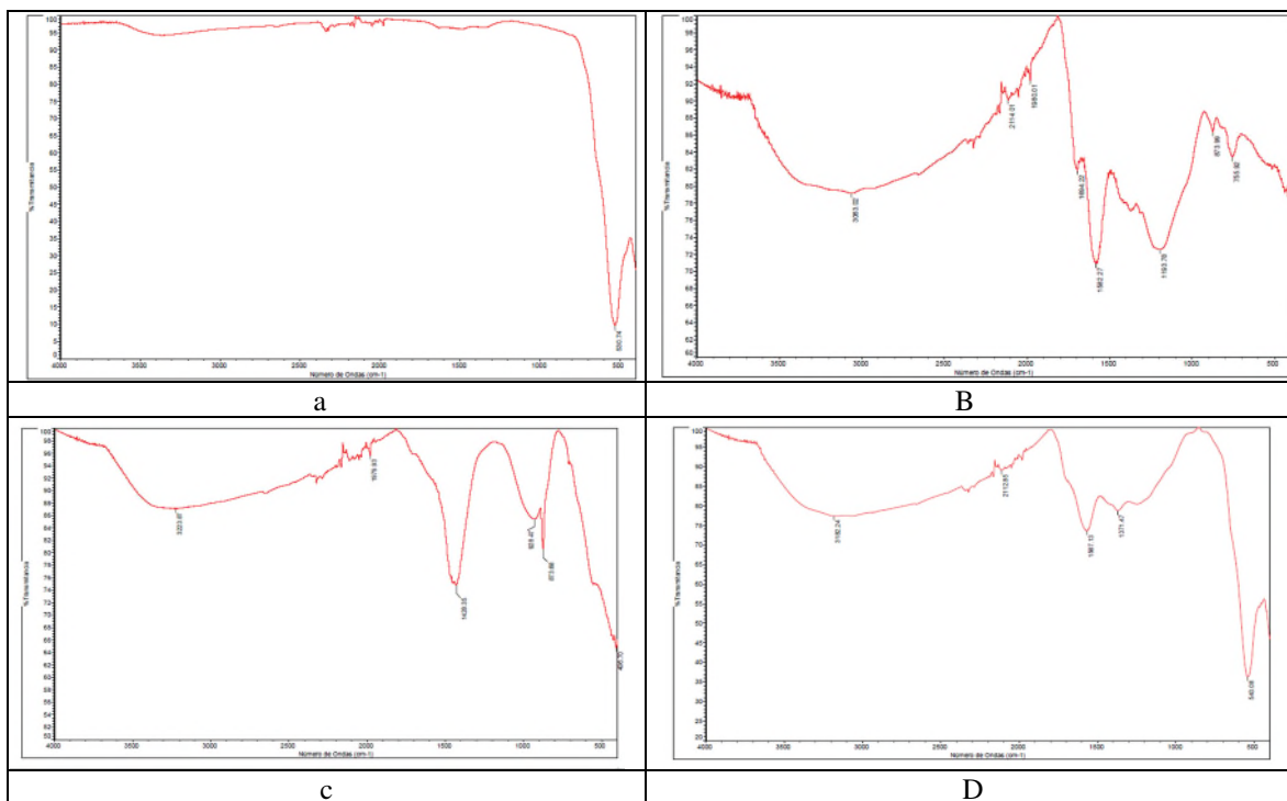
Figura 4. FTIR spectra: a) MNP, b) biochar, c) BMNP, d) MM
