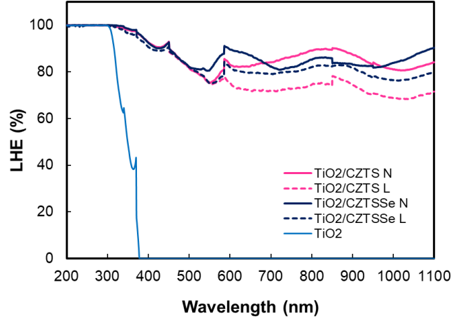
Figure 10. Light harvesting efficiency of solar cells CZTS N, CZTS L, CZTSSe N, CZTSSe L, TiO 2
