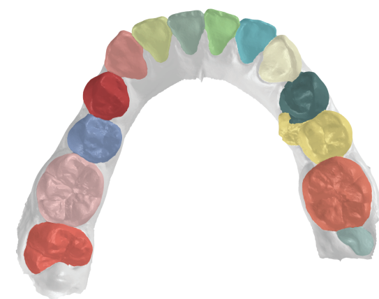
Case 10. DC-Net
