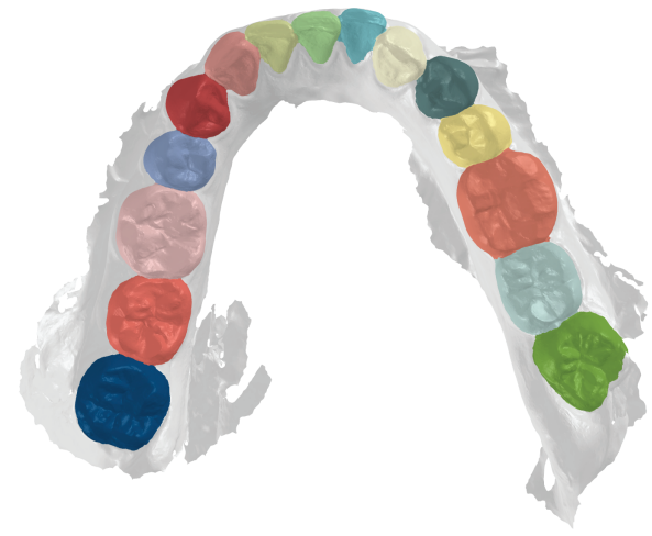
Case 10. DC-Net
