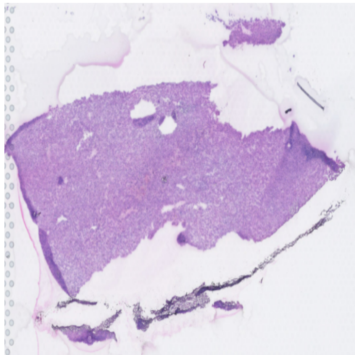
MIF ligand
