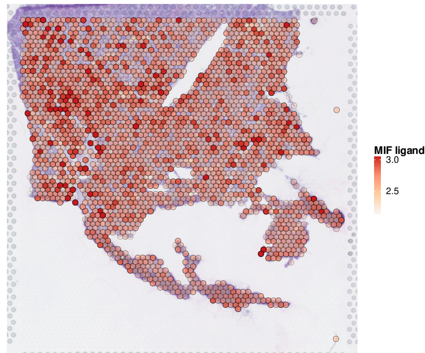
MIF ligand
