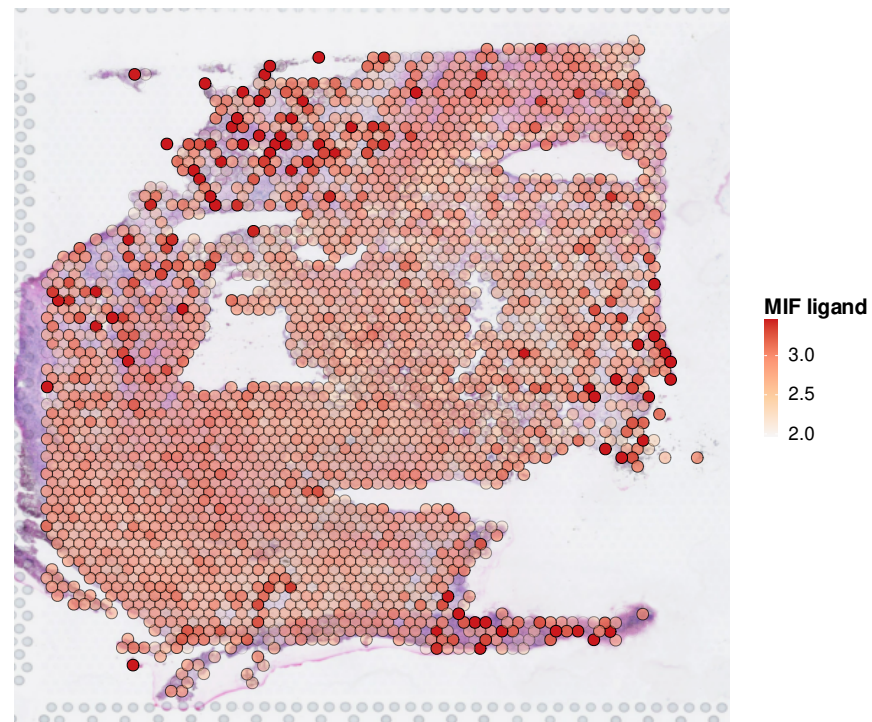
MIF ligand
