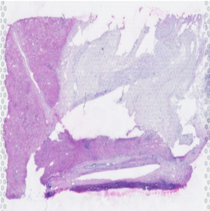
MIF ligand
