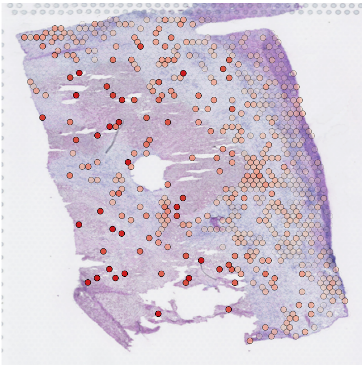
MIF ligand
