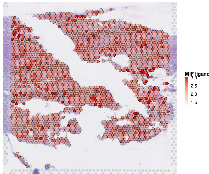
MIF ligand
