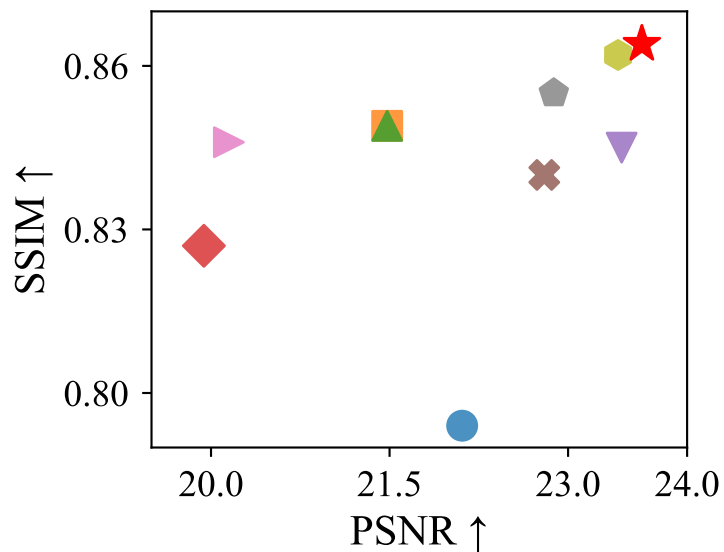
LOL-V2-Real
