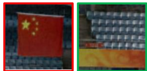
SNR
