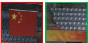
CIDNet
